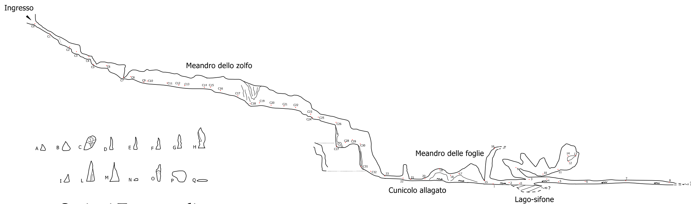
Sezioni Trasversali
